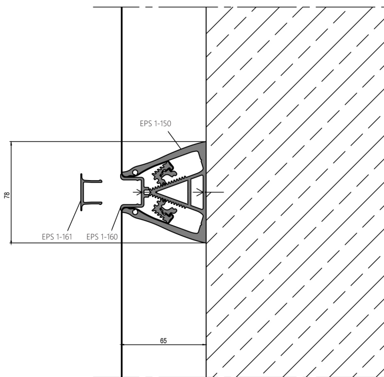
Befestigung auf mineralischem Untergrund
