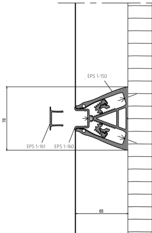
Befestigung auf Holz
