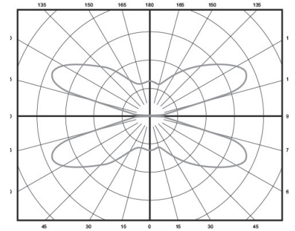
Lichtstärkeverteilung
