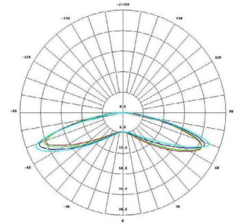
Lichtverteilung
