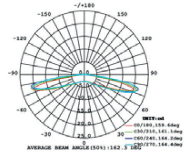
Lichtverteilung
